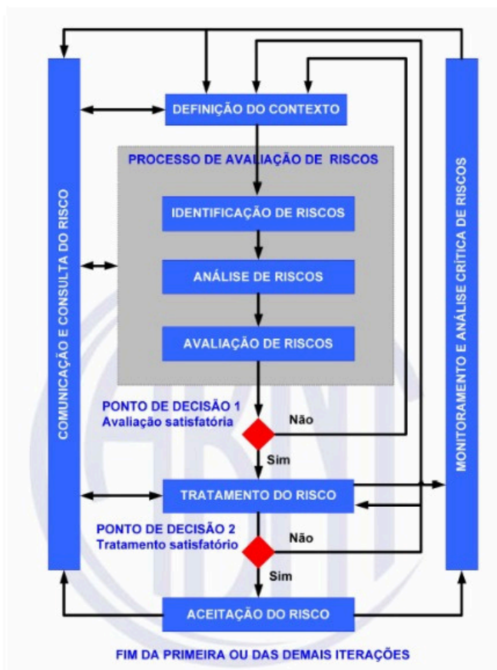
Figura 5: O processo de Gestão de Riscos de TIC – Fonte: ABNT NBR 27005:2019
